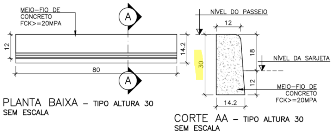
Figura 11 - Detalhe do meio-fio. Elaboração própria. Nota: Desenho elaborado em 12/12/2019
